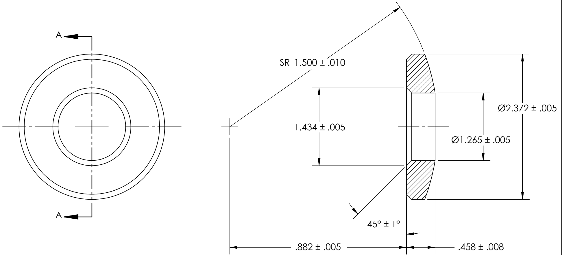
SECTION A-A
